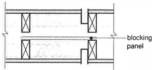
a) Plan
