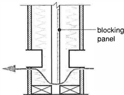
b) Section
