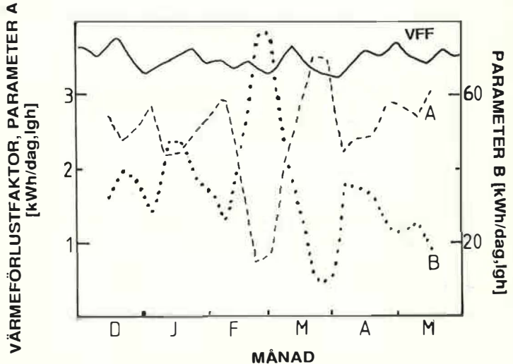
Fig. 7 Stabilitet av beräknad Värmeförlustfaktor (VVF) jämförd med stabilitet av energisignaturparametrar A och B. Angivna värden är baserade på 7 mättdagar (VVF) respektive 28 mättdagar (energisignatur). Data för flerf.hus # 1.
