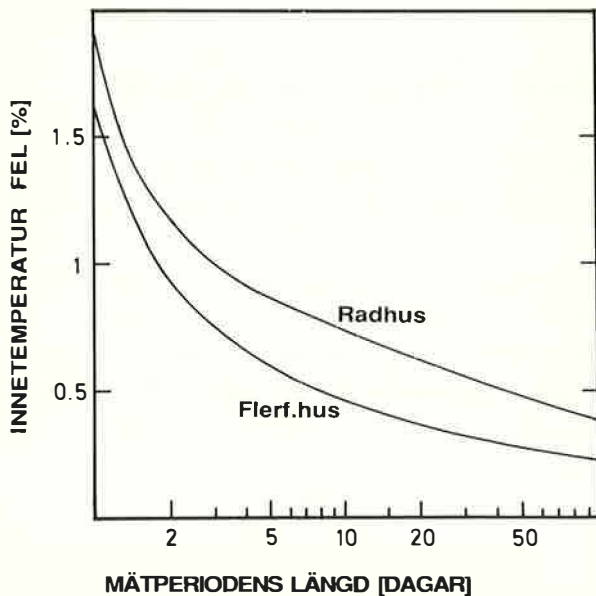
Fig. 13 Medelfel i förutsagd innetemperatur under eldningsäsongen från kortidsmätningar.
