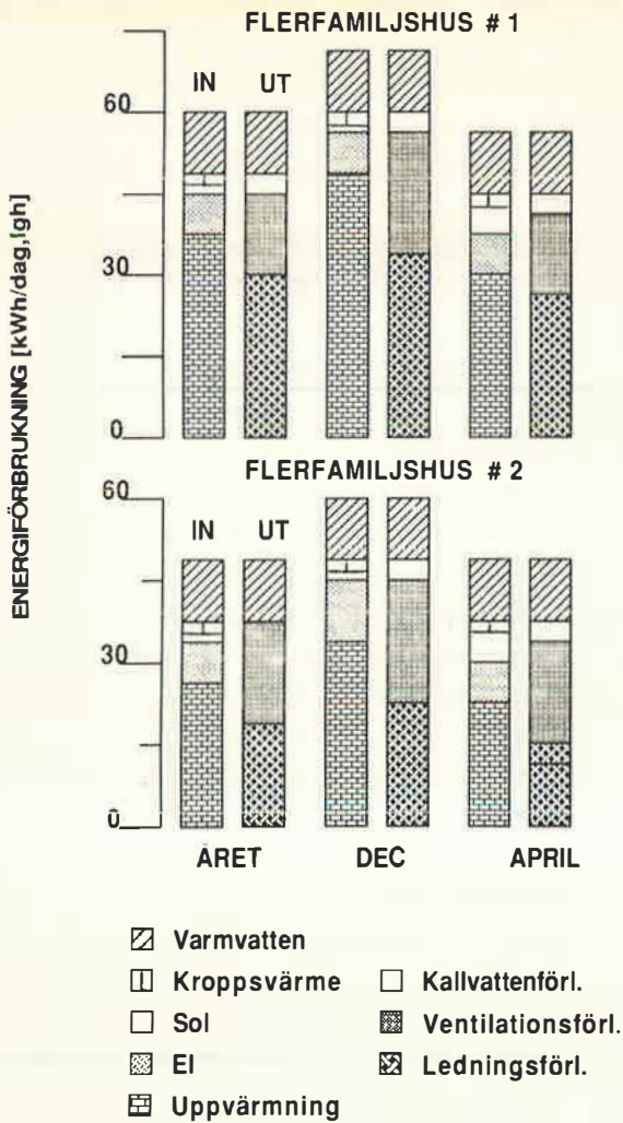
Fig. 14 Energibalans för de studerade flerfamiljshusen för april, december och för eldningsårssongen
