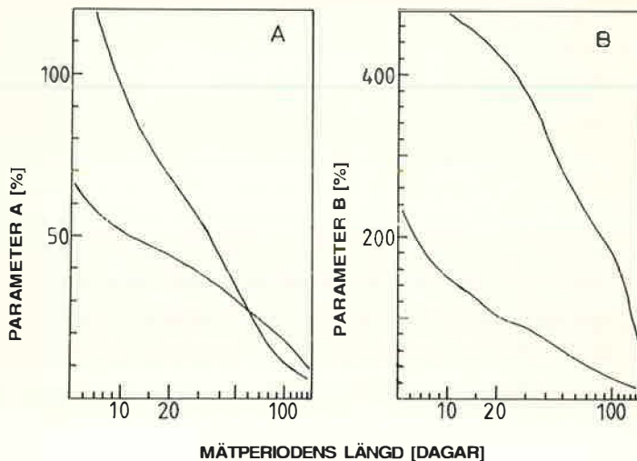
Fig. 8 Medelfel (en standardavvikelse) i förutsägelse av årligt värde av energisignaturparametrar A (vänster) och B (höger) från kortidsmätningar.
