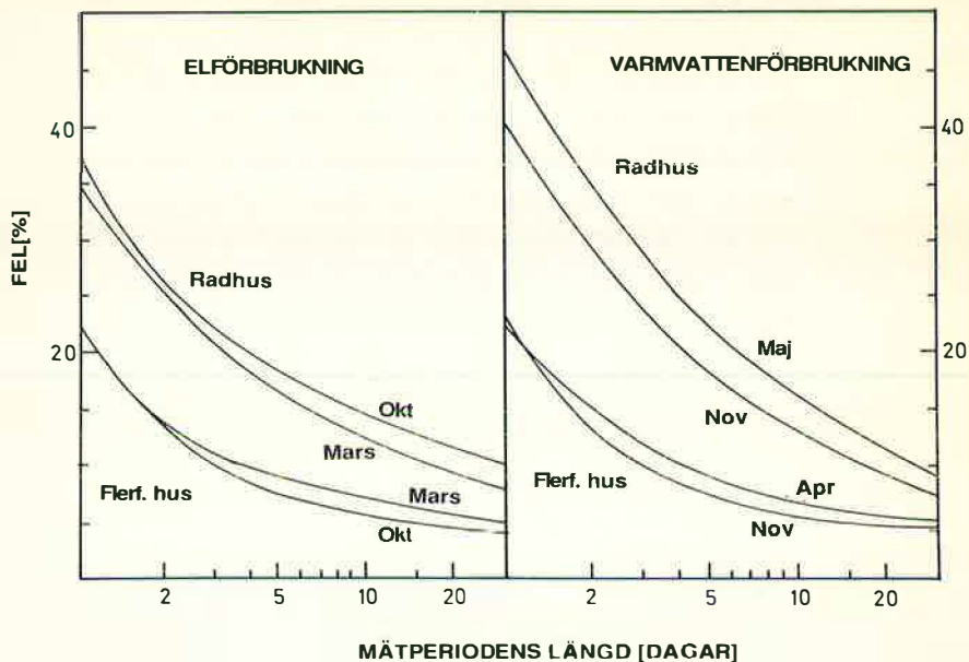
Fig. 12 Medelfel (en standardavvikelse) i förutspådd årsförbrukning av el (vänster) och varmvatten (höger) från korttidsmätningar under månader med medelförbrukning nära årsmedelförbrukning.
